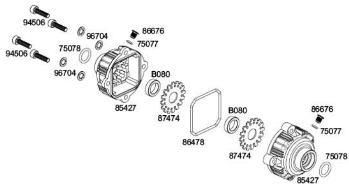
85427 ALLOY DIFFERENTIAL CASE SET ALUMINIUM DIFFERENTIALGEHAEUSE SET JEU BOITIER DE DIFFERENTIEL ALLIAGE メタルデフケースセット
